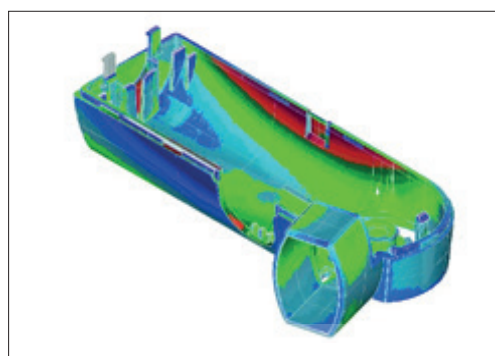
Inhalateur - comparaison pièce/CAO avec colorimétrie
